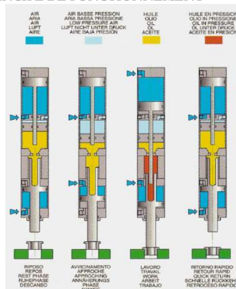
Figure n.2 _ Principe de fonctionnement
