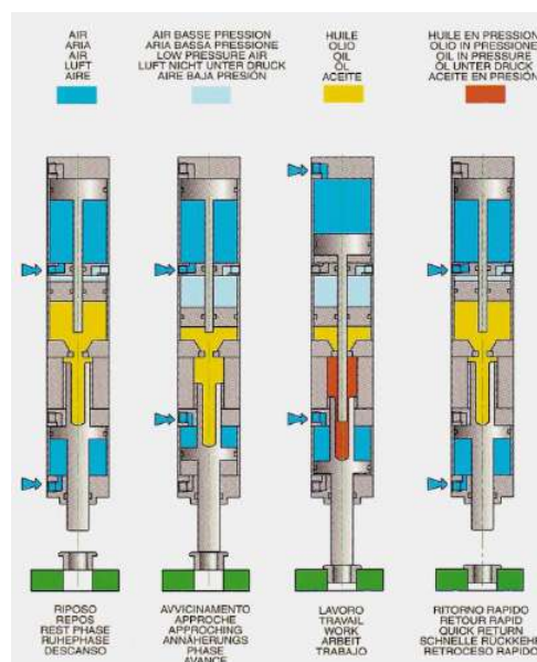
Rysunek 2_Zasada działania
