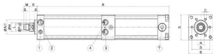
Rysunek 1 _ schemat siłownika
