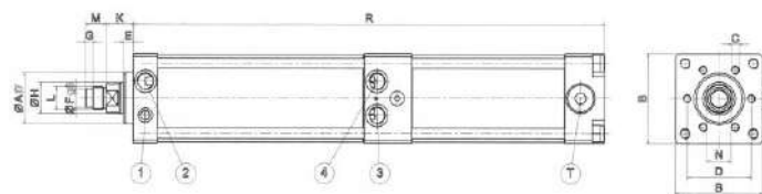
Figure 1 _ Vue unité et orifices
