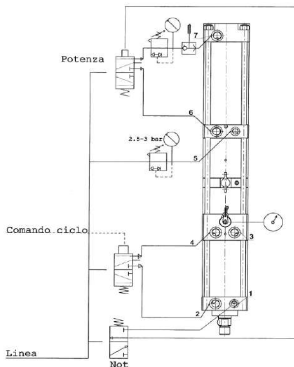
Figure 3 – Schéma pneumatique de référence_version « E »
