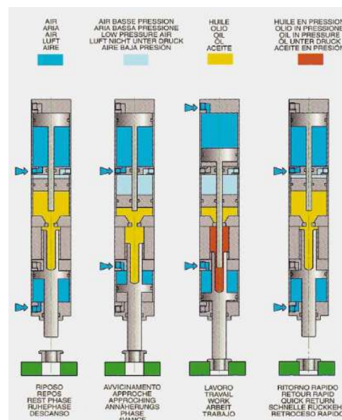
Abbildung 2 _ Betriebsprinzip
