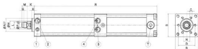
Figura 1 _ vista schematica unità
