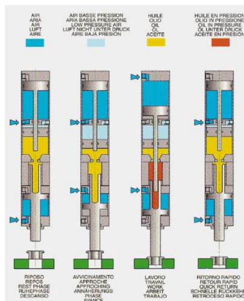
Figura 2 _ principio di funzionamento
